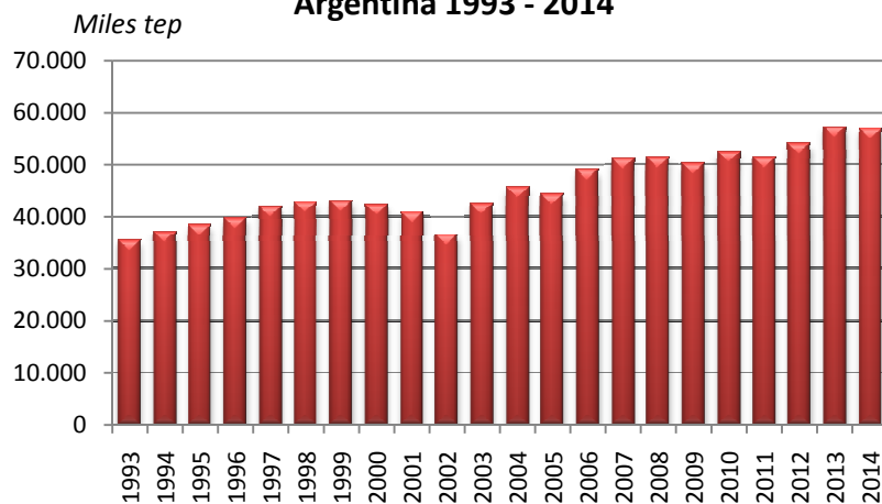
Evolución del consumo de energía Argentina 1993 - 2014
