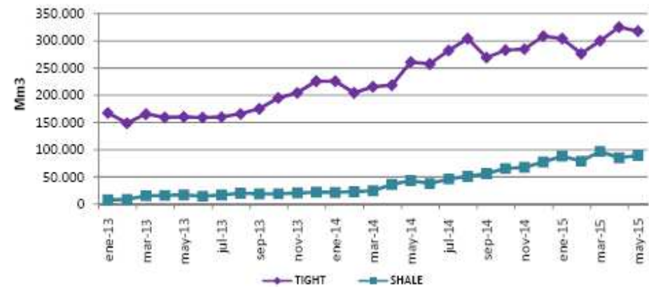
Producción de gas no convencional
