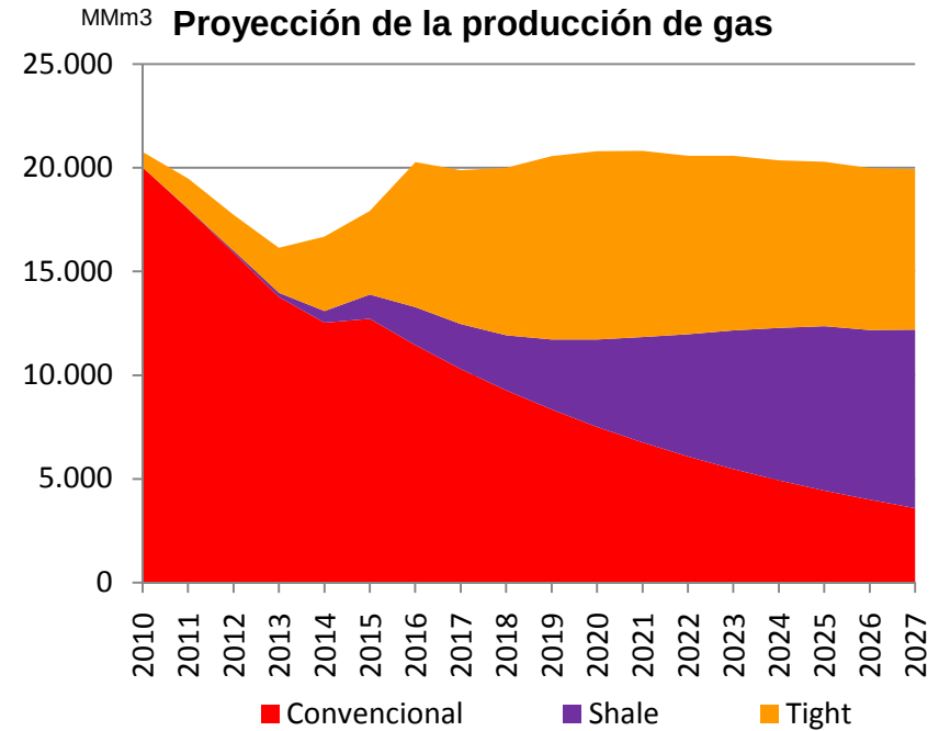
Producción de gas no convencional
