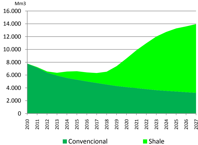
Proyección de la producción de petróleo
