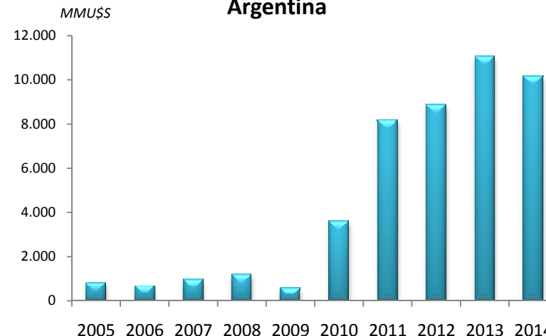
Evolución de las importaciones de energía Argentina
