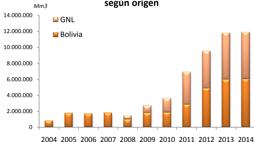
Evolución de las importaciones de Gas Natural según origen
