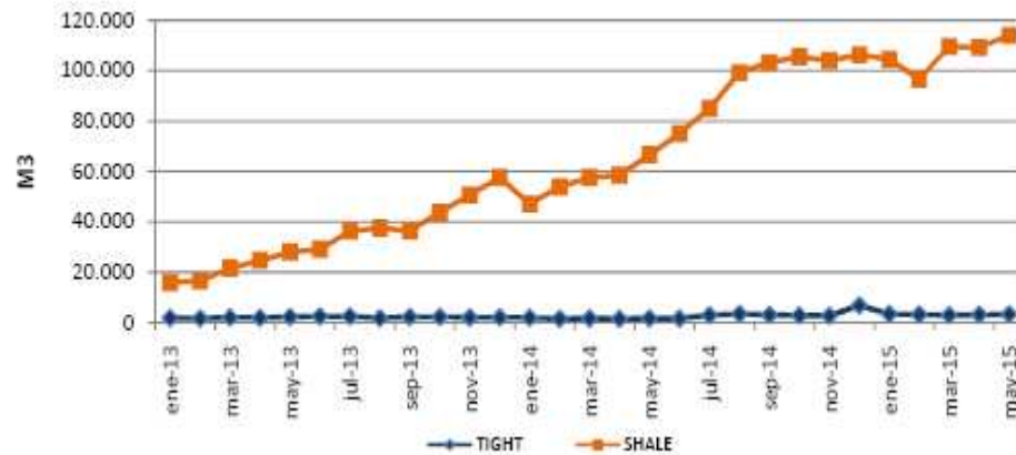
Producción de petróleo no convencional
