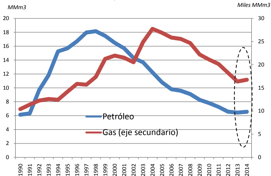
Evolución de la producción de petróleo y gas Neuquén 1990 - 2014
